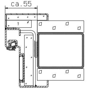
bekleidetes Stahlprofil
